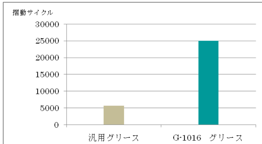
グラフ 1 : 亜鉛メッキ上での潤滑寿命試験
