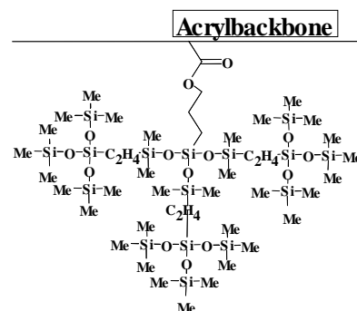
トリメチルシリル基(Me 3 Si)を、規則的な球状に配したデンドリマー構造
